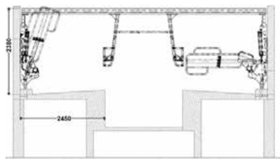
Vue de coupe ECS 700 Fast Exit..
